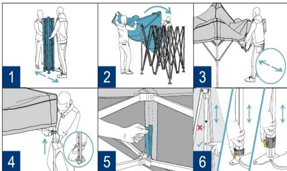
Rys.2 Przebieg montażu namiotu ekspresowego
